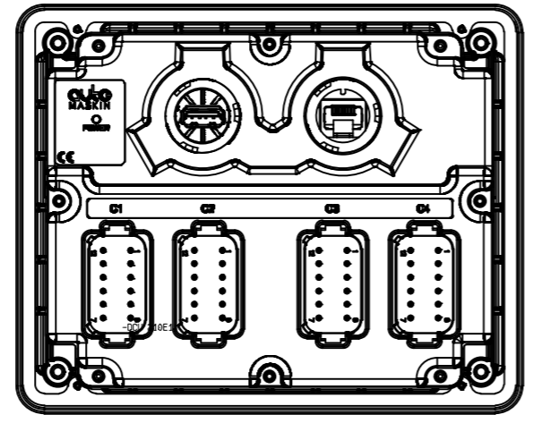
DCU 210E BACK
